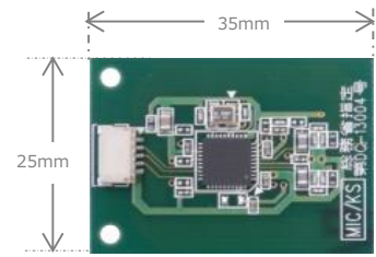
(ARI3030 外観)
